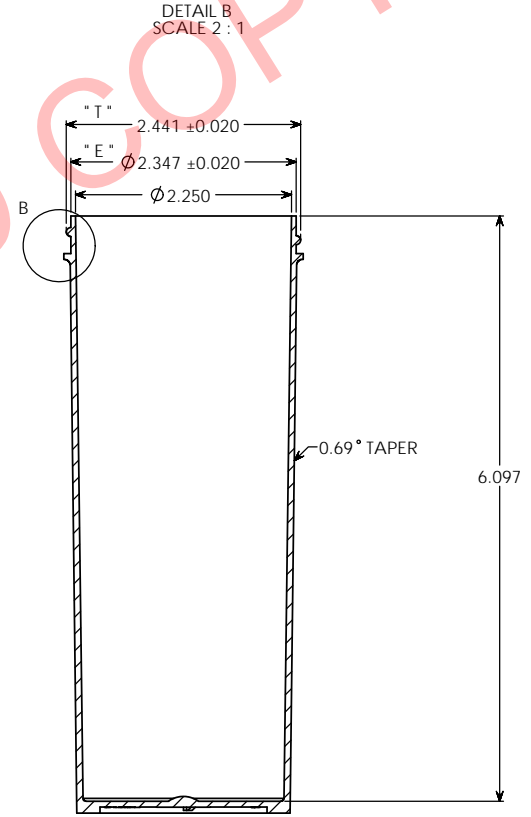
SECTION A-A
