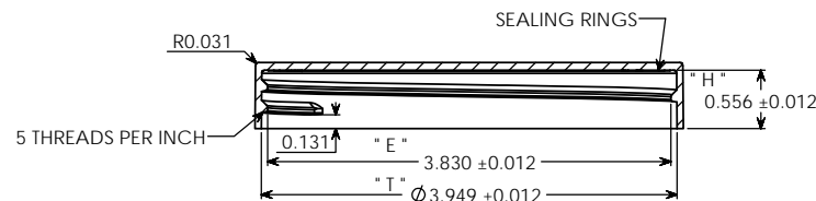
SECTION A-A
